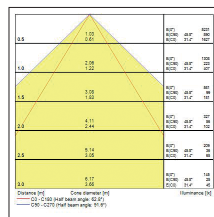
Prismatisch
