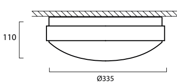
Giotto LED G2 335 En saillie
