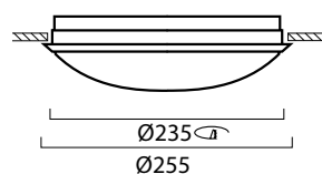
Giotto LED G2 235 Encastré
