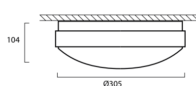
Giotto LED G2 305 En saillie
