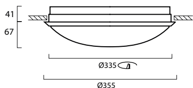
Giotto LED G2 335 Encastré
