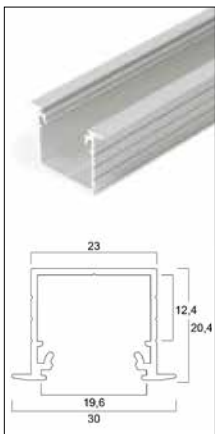
Inbouwprofiel 20 EF/U7
