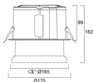
STANDARDVERSION, MIT FLANSCH
