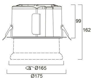
VERSION TL, OHNE FLANSCH
