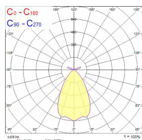
NICHT AUSGEFAHRENE OPTIK
