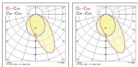
Raxa Wallwasher 900 3000K
