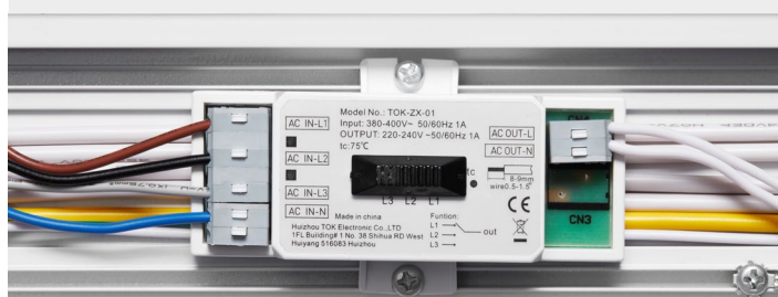
Fase-keuzeschakelaar
