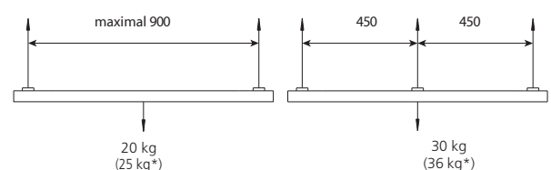
Maximale Belastung
