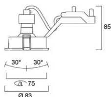
Inset Trend SW IP23
