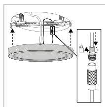
Half-inbouw installatie
